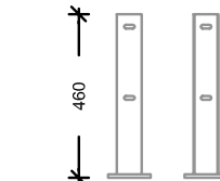
Supporto di ancoraggio
